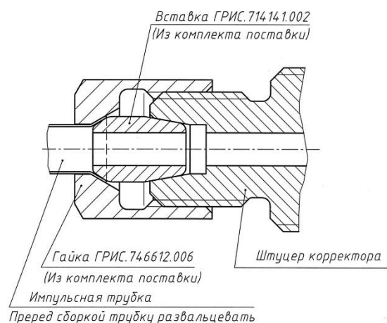
Рисунок 18 – Рекомендоване підключення імпульсної трубки до штуцеру корректора
