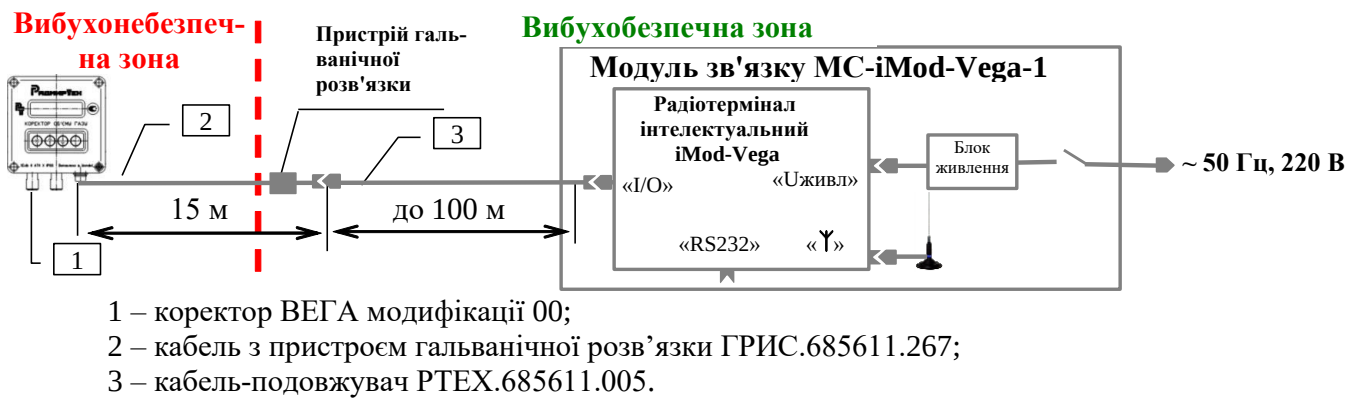
Рисунок 49 – Схема підключення модуля зв'язку MC-iMod-Vega-1
