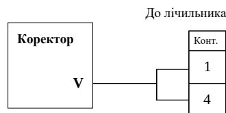
Рисунок 21 – Схема розпайки кабелю коректора до лічильника газу типу ЛГ
