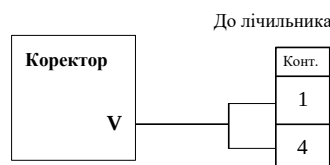
Рисунок 23 – Схема розпайки кабелю коректора до лічильника газу типу Schlumberger
