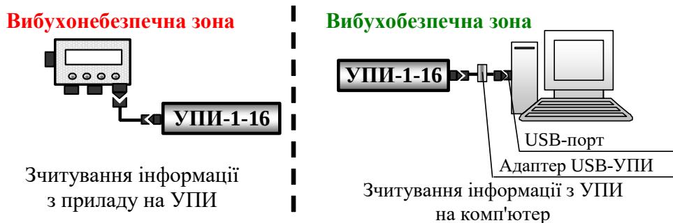
Рисунок 40 – Зчитування інформації з коректорів ВЕГА модифікації 00 за допомогою УПІ-1-16
