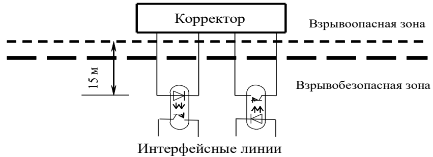
Рисунок 8 – Функціональний вузол, що забезпечує вибухозахищеність коректора
