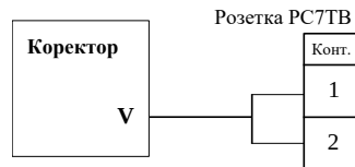
Рисунок 25 – Схема розпайки кабелю коректора до лічильника газу типу «ТЕМП»
