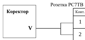
Рисунок 20 – Схема розпайки кабелю коректора до лічильника газу типу РГ
