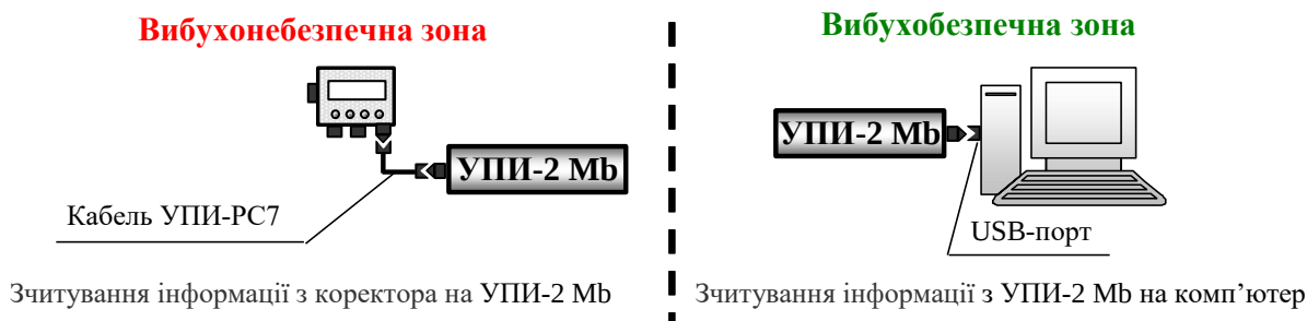
Рисунок 38 – Зчитування інформації з коректорів ВЕГА модифікації N0 за допомогою УПІ-2Мб
