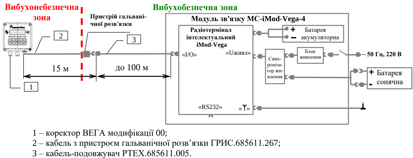
Рисунок 50 – Схема підключення модуля зв'язку MC-iMod-Vega-4
