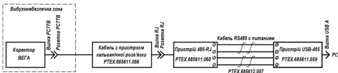
Рисунок 46 – Двосторонній зв'язок коректорів ВЕГА з можливістю передачі даних на великі відстані (до 1000 м)
