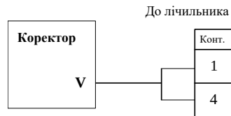
Рисунок 24 – Схема розпайки кабелю коректора до лічильника газу типу GMS
