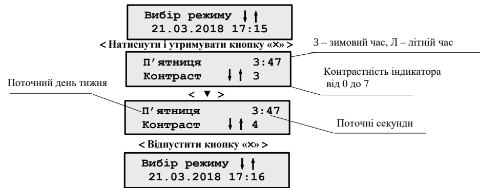
Рисунок 10 – Регулювання яскравості індикатора
